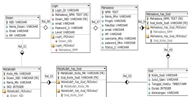
Gbr. 6 EER sistem ujian online berbasis SMS
