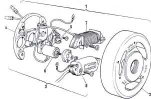
Gambar 7 Contoh konstruksi Flywheel Generator(Jalius Jama Wagino, 2008)
