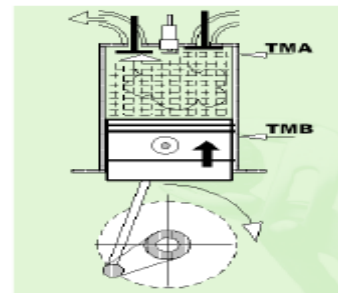
Gambar 1. Batas TMA dan TMB piston (Jalius Jama Wagino, 2008) □
