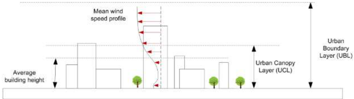
Gambar 1. Profil lapisan angin daerah urban [14]
