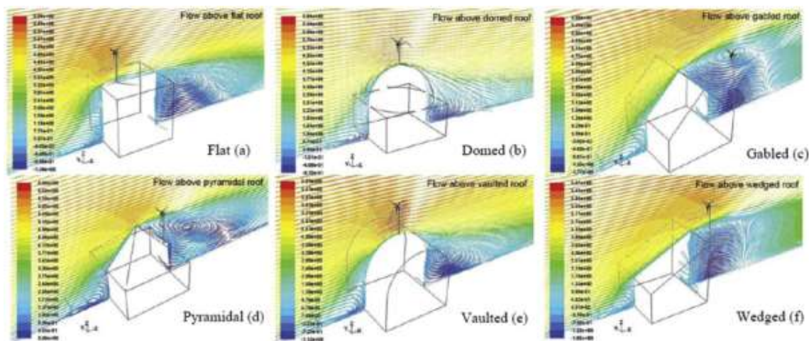
Gambar 2. Macam-macam Rooftop Profil dan bentuk arah-aliran angin [15]
