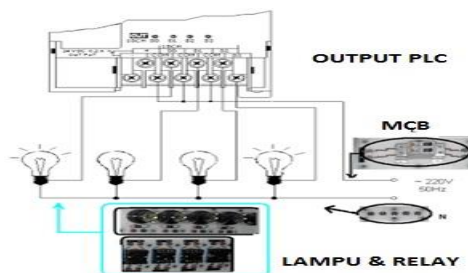
GAMBAR 3 PENGAWATAN OUTPUT
