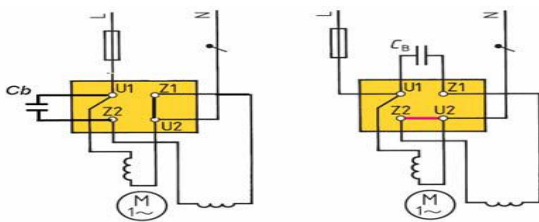
Gambar 2. Cara sambungan membalikan motor 1 phase
