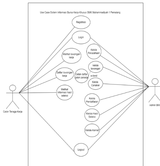
Gambar 1 Use Case Sistem Informasi Bursa Kerja Khusus SMK Muhammadiyah 1 Pemalang
