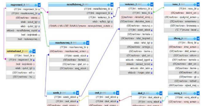
Gambar 3 Gambar Class Diagram Sistem Informasi BKK SMK Muhammadiyah 1 Pemalang
