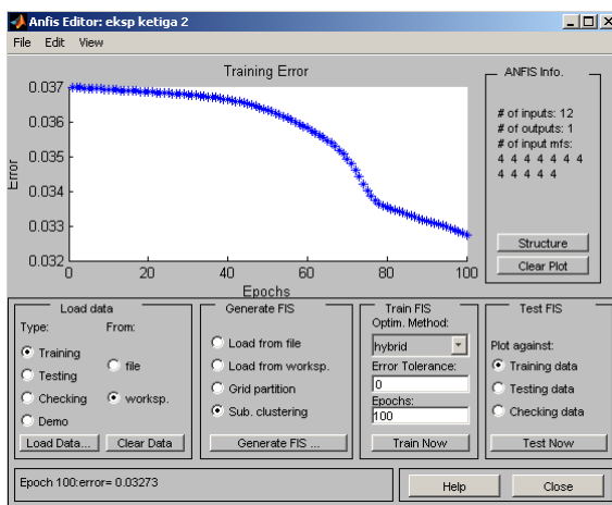
Gambar 4. Hasil Error Toleransi eksperimen 5
