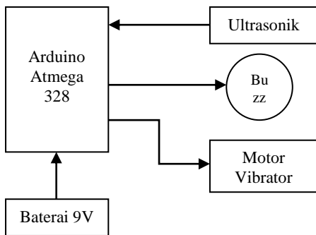
Gambar 1. Diagram Blok Smart Blind Stick dengan Atmega 328
