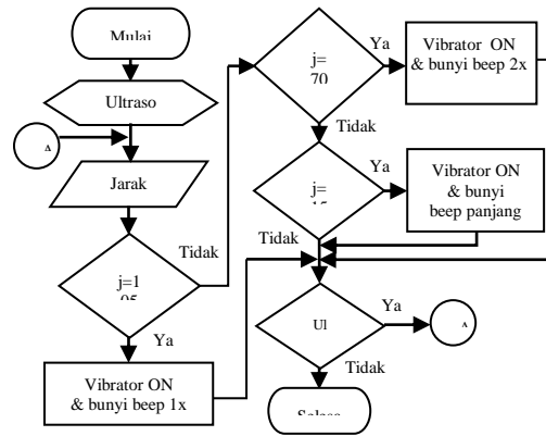
Gambar 2. Diagram Alir Smart Blind Stick dengan Atmega 328
